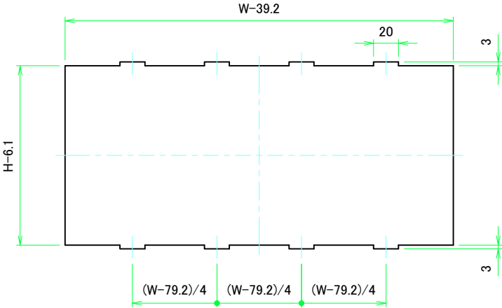
Wパネル1表面 / W Panel 1 Frontside
