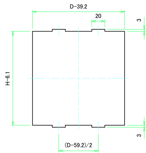
Dパネル1表面 / D Panel 1 Frontside
