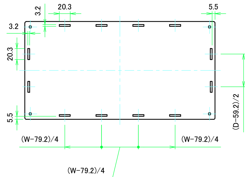
上カバー裏面 / Top cover Backside
