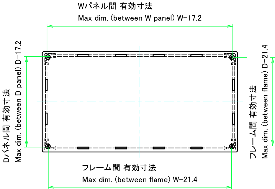
下カバー / Bottom cover
